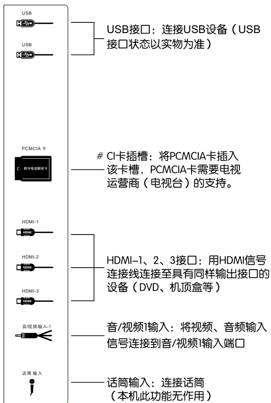
AV端子右示意图
