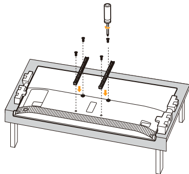
3 用挂架螺钉把挂架锁到电视整机上
