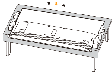
2 将VESA塑胶转接柱放到VESA孔处
