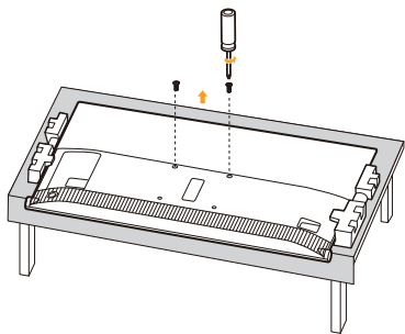
1 从后壳上取下VESA螺钉
