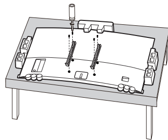
3 用挂架螺钉把挂架锁到电视整机上
