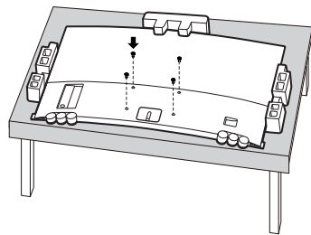
2 将VESA塑胶转接柱放到VESA孔处
