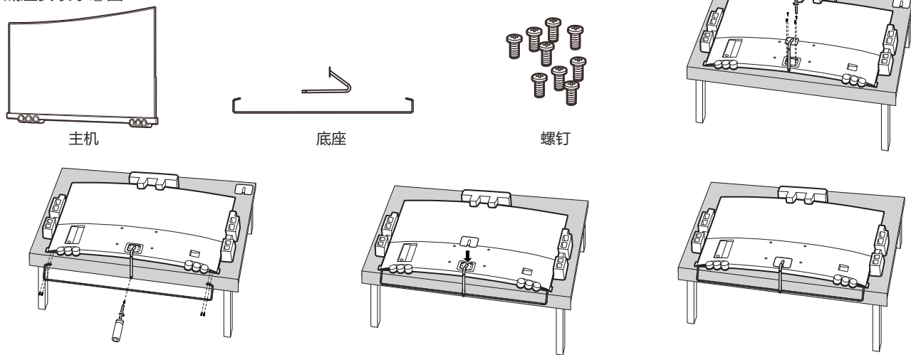
底座安装示意图
