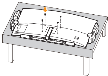
8 将VESA塑胶转接柱放到VESA孔处
