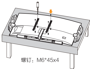
9 用挂架螺钉把挂架安装到电视整机上
