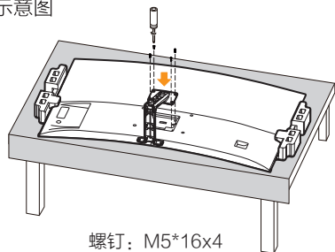
底座安装示意图
