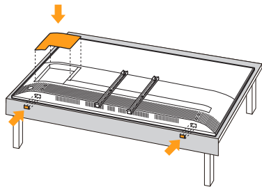
④ 将AV端子盖板从附件袋中取出，插好线材，如图所示将AV盖板固定在电视机相应位置；然后将底座盖板从附件袋中取出，如图所示将底座盖板装好。
