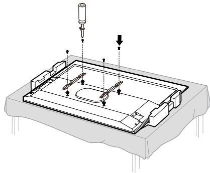
2、先装上四个VESA转接支架，再装挂架，然后用挂架螺钉把挂架锁到电视整机上。
