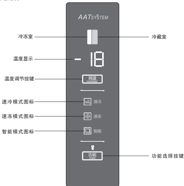
图示为BCD-518WEPF1电脑控制面板
