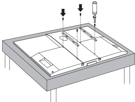
② 用后壳取下的4颗VESA螺钉将挂架锁到电视整机上
